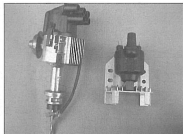
Electronische ontsteking
